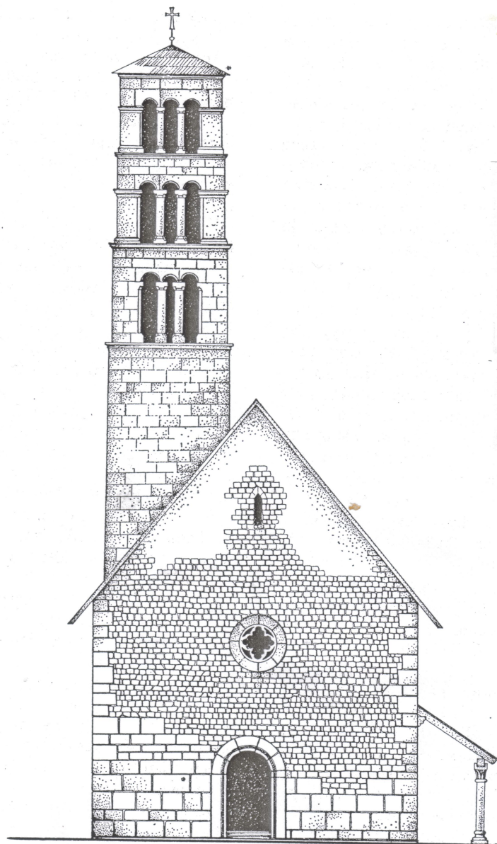
Sl. 51. JAJCE – pročelje crkve sv. Marije. Stanje u XV stolj.
