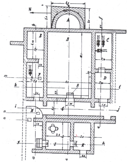
Lepenica: Tlocrt crkve (prema Skariću)
